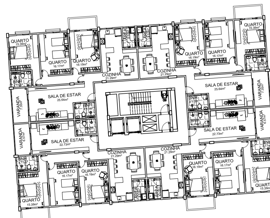
4 PLANTA PAVIMENTO TIPO MODELO 3 ESCALA 1/250
