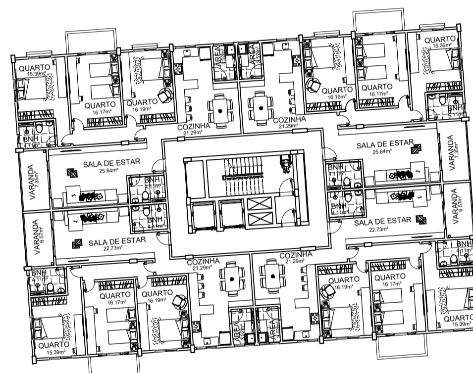
3 PLANTA PAVIMENTO TIPO MODELO 2 ESCALA 1/250
