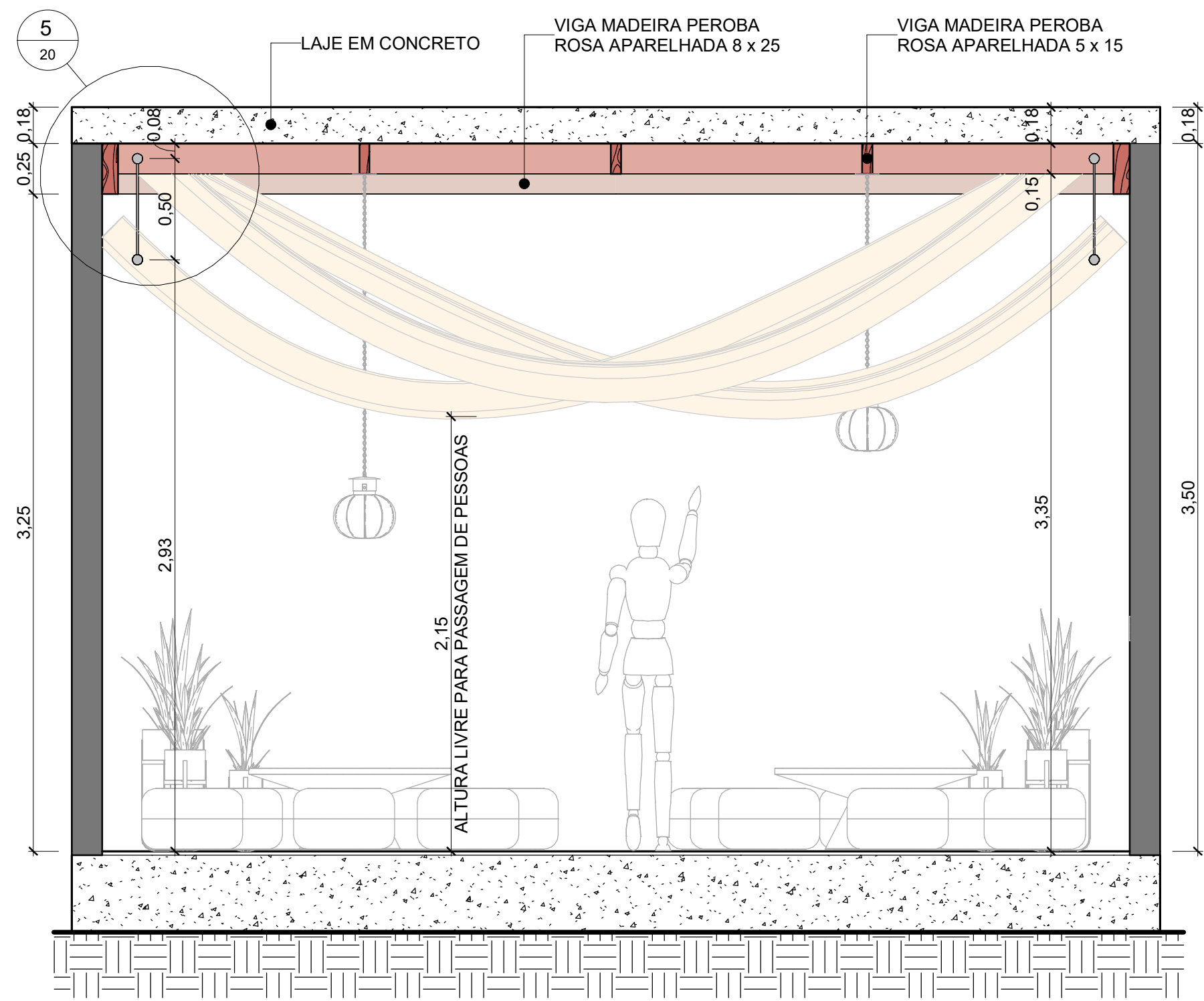
1 CORTE AA - SALÃO PRIVATIVO 1 : 25
