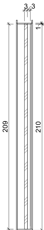
6 P06 - CORTE 1 : 20
