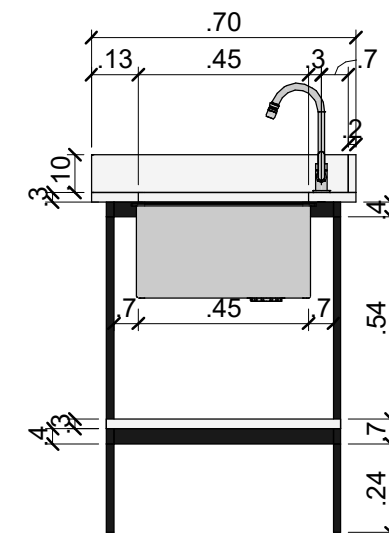
7 BG4: CORTE 1 : 20
