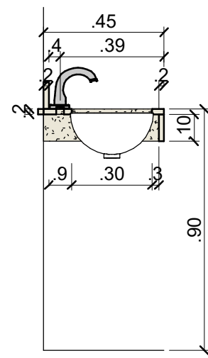
7 BG2: CORTE 1 : 20
