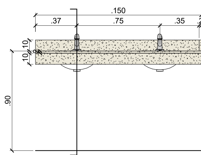
2 BG1: VISTA FRONTAL 1 : 20
