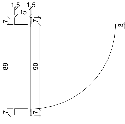
8 P03 - PLANTA 1 : 20
