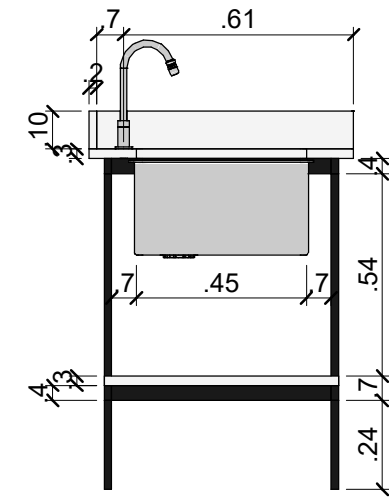
3 BG3: CORTE 1 : 20
