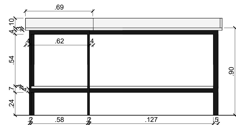
3 BG5: CORTE 1 : 20
