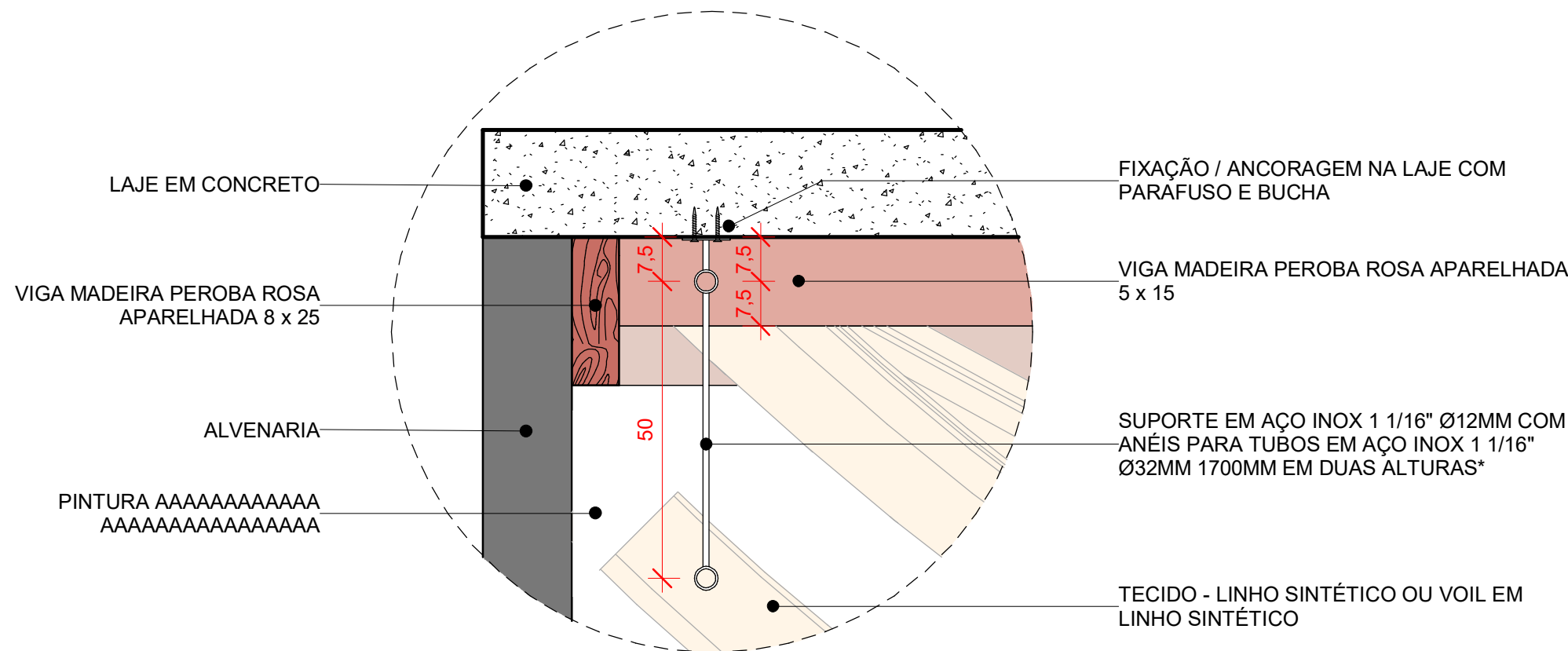
1 CORTE AA - SALÃO PRIVATIVO 1 : 25
