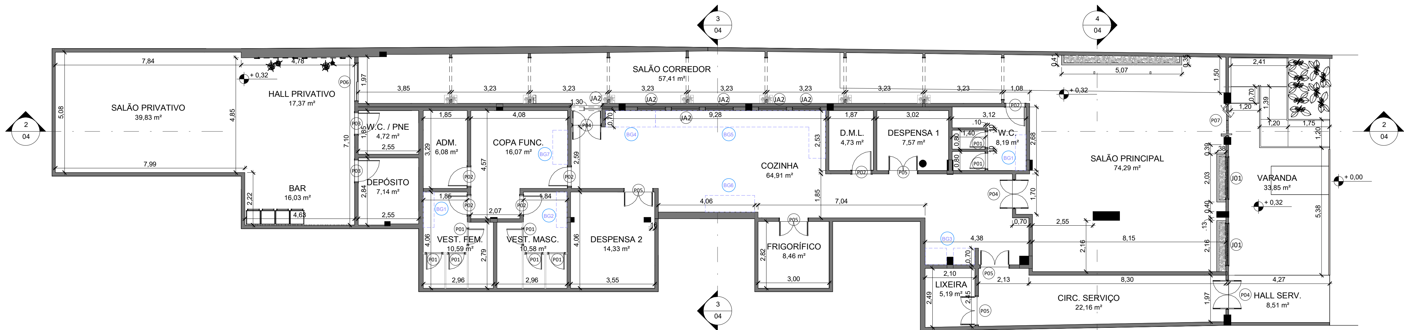
1 PLANTA ARQUITETURA 1 : 100
