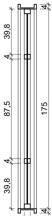
8 J01 - PLANTA 1 : 20
