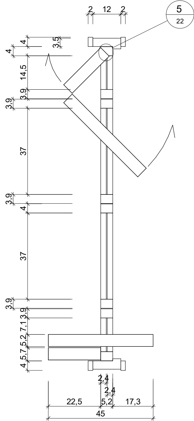
4 PLANTA - P07 1 : 10
