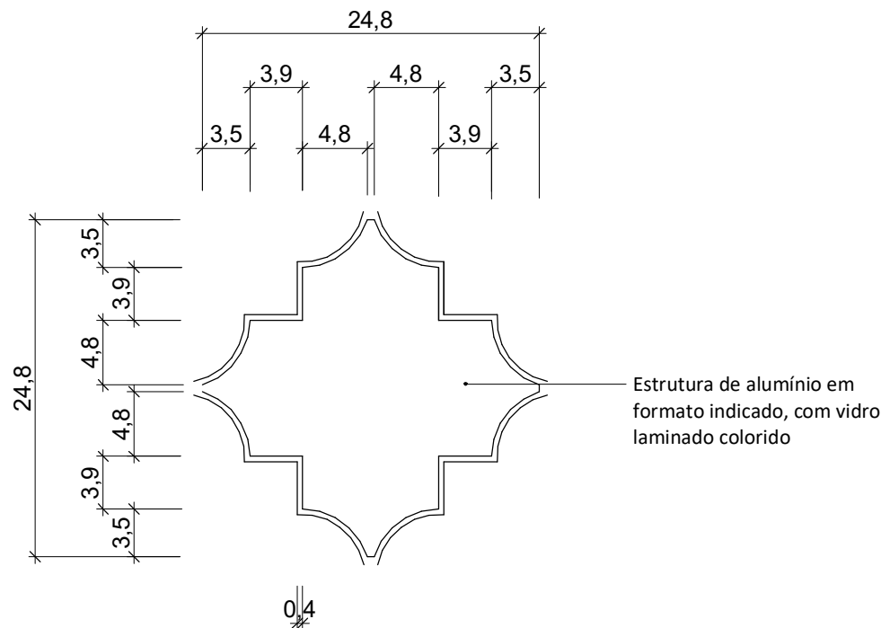
4 PLANTA - P07 1 : 10
