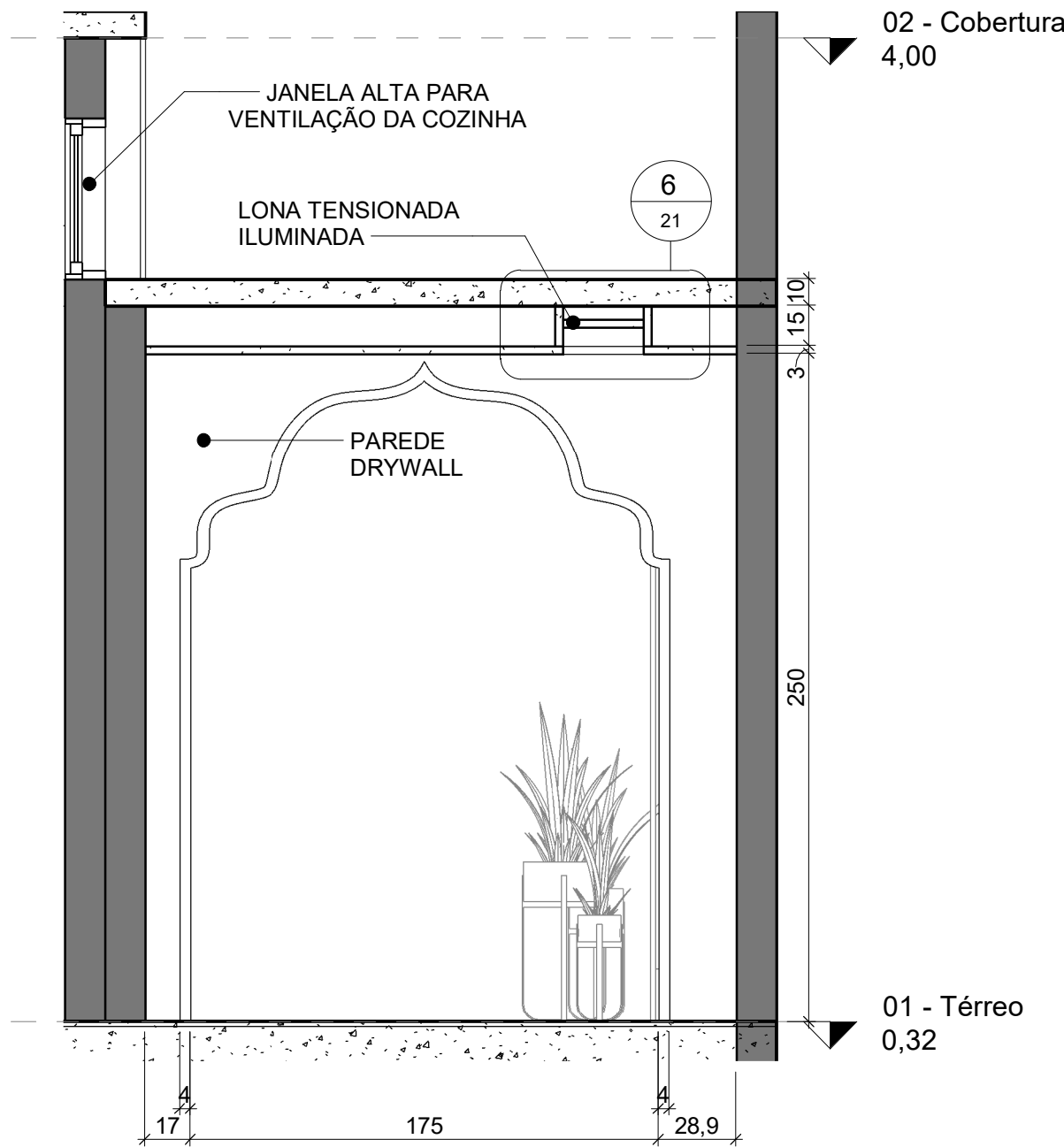
1 VISTA - PAREDE DRYWALL 1 : 25
