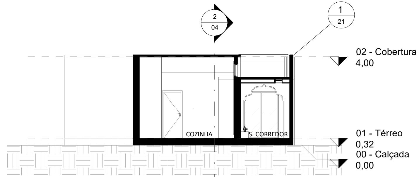
3 CORTE DD 1 : 100
