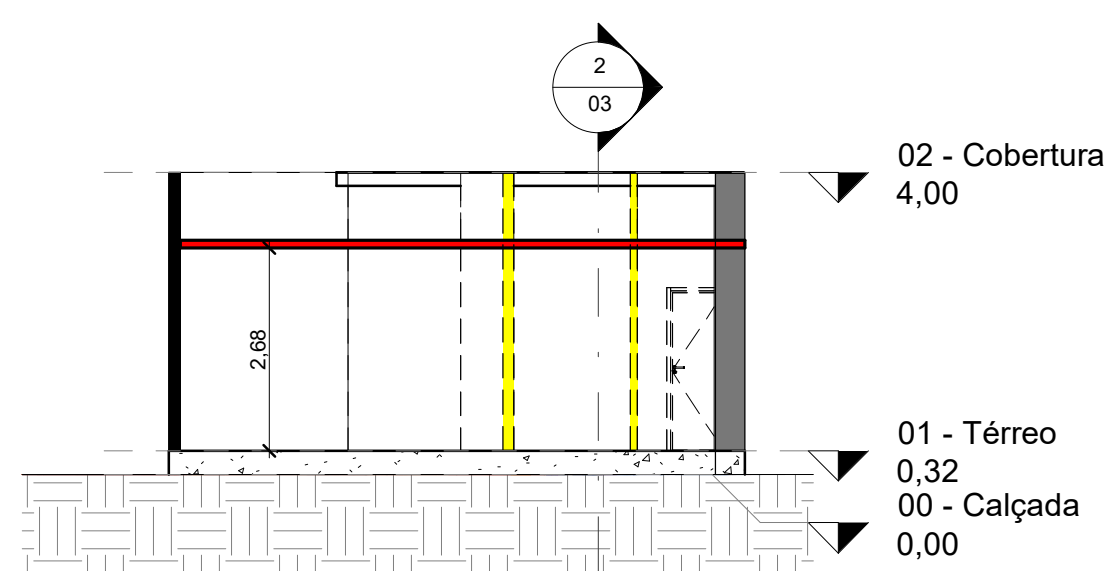
3 CORTE BB 1 : 100
