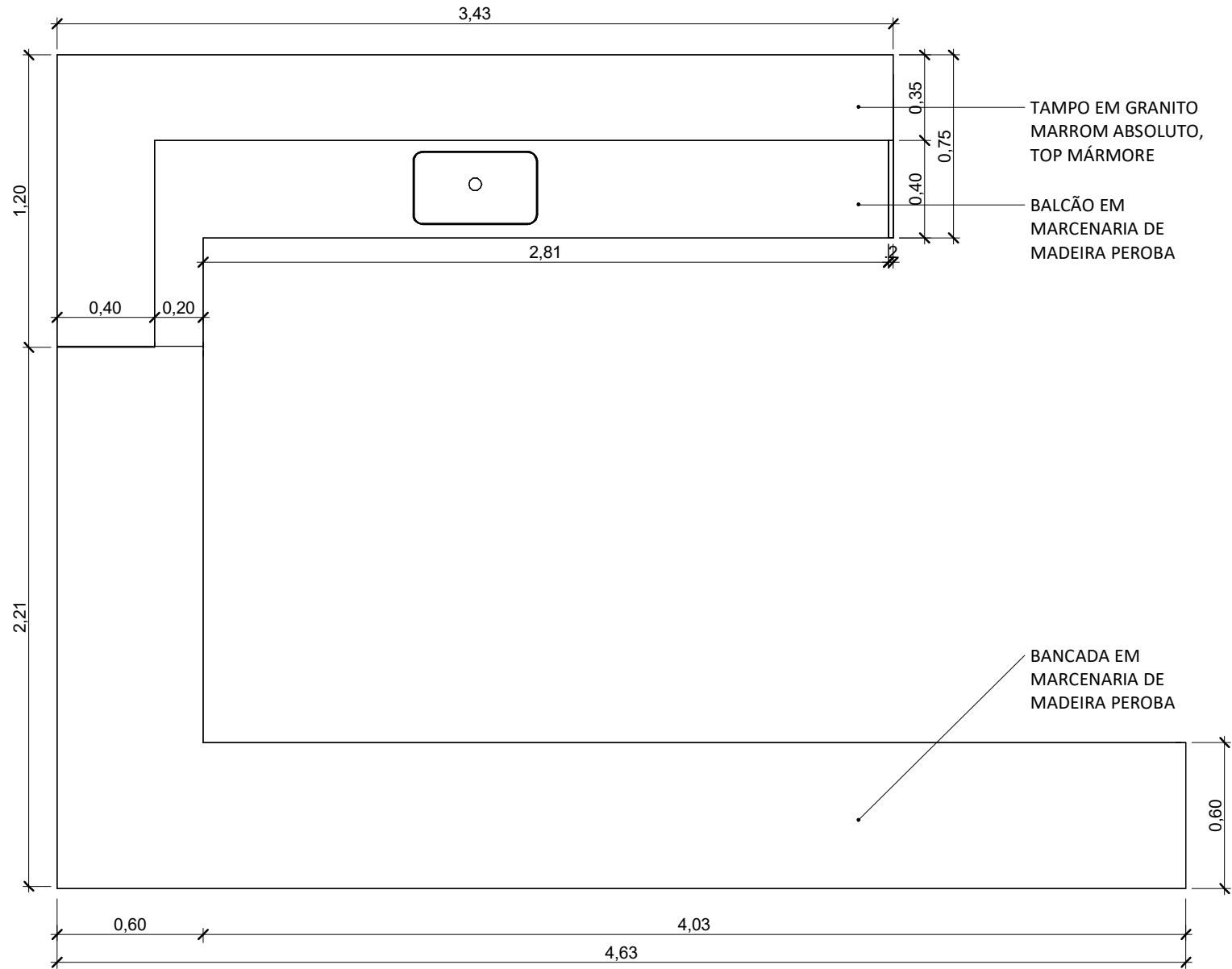
1 PLANTA BANCADA BAR 1 : 25
