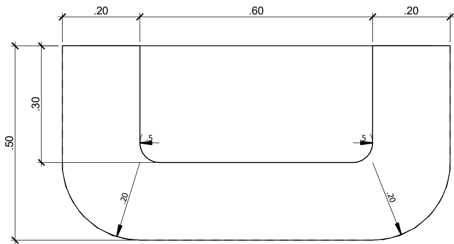
1 PLANTA BANCADA RECEPÇÃO 1 : 10
