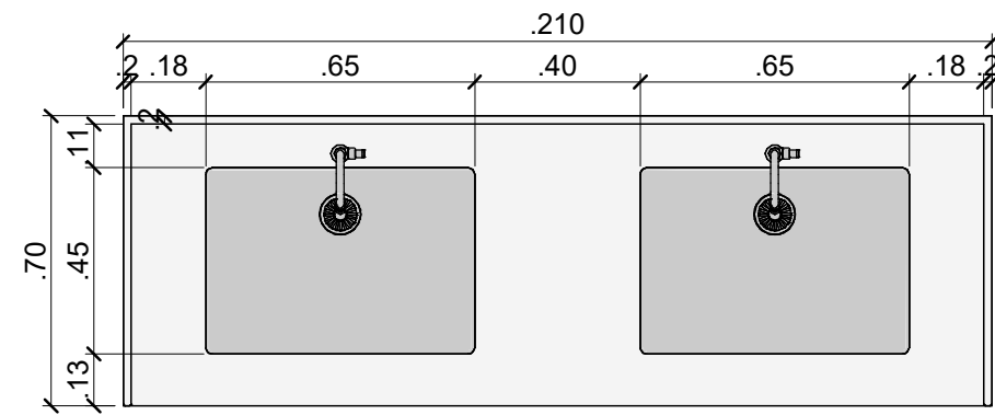
5 BG4: PLANTA 1 : 20
