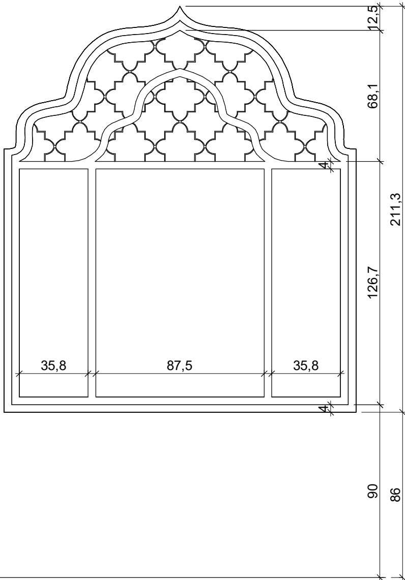
7 J01 - VISTA FRONTAL 1 : 20
