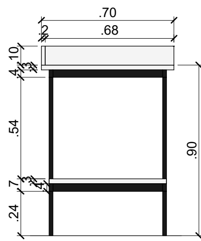
3 BG6: CORTE 1 : 20
