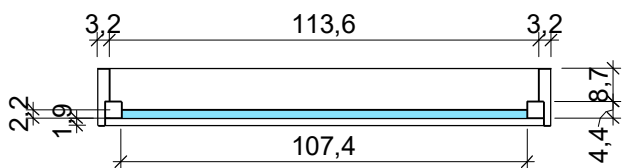
11 J02 - PLANTA 1 : 20
