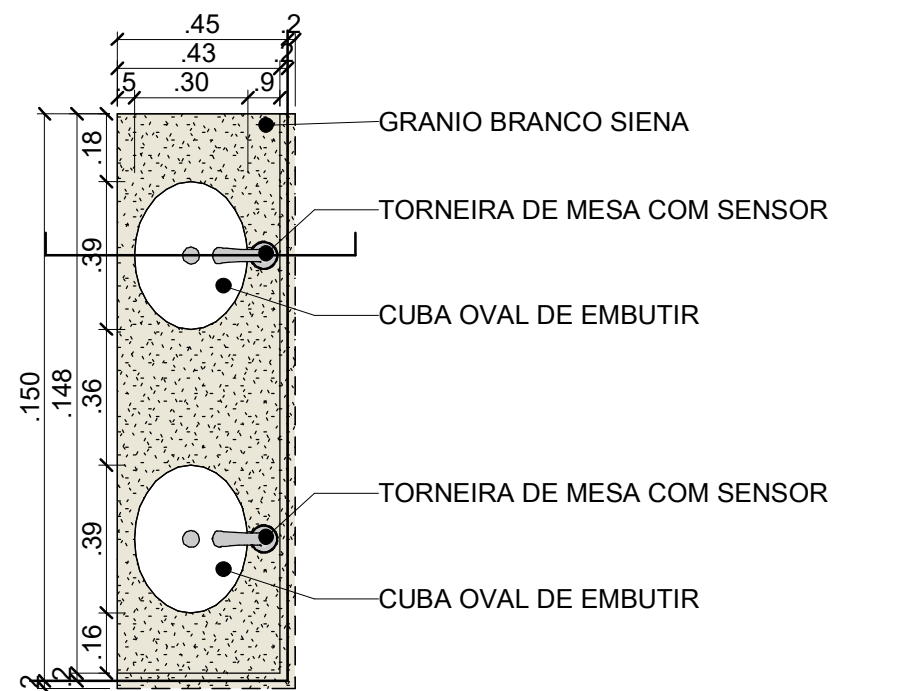
1 BG1: PLANTA 1 : 20
