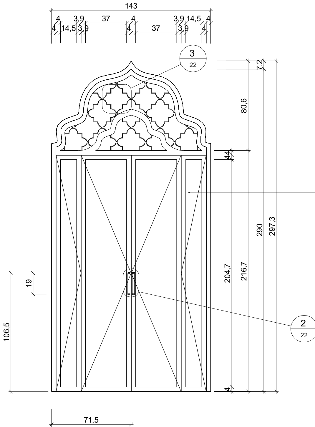
1 ELEVÇÃO FRONTAL 1 : 20
