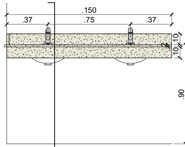
6 BG2: VISTA FRONTAL 1 : 20
