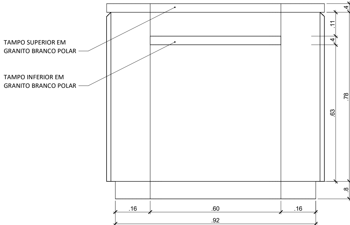
4 ELEVÇÃO POSTERIOR 1 : 10
