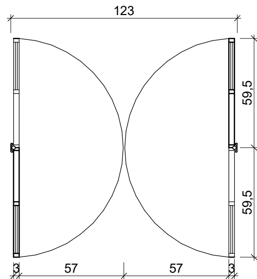
11 P04 - PLANTA 1 : 20
