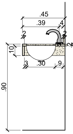
3 BG1: CORTE 1 : 20
