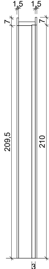
9 P03 - CORTE 1 : 20
