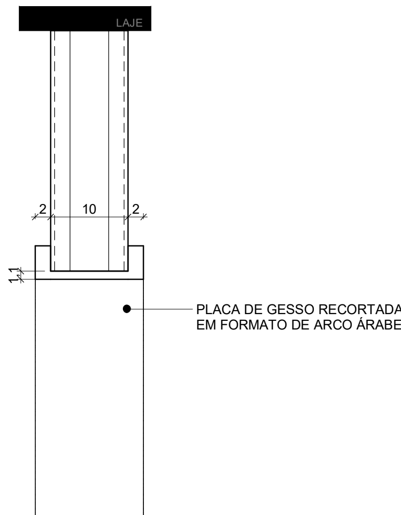
5 DETALHE D - CORTE MOLDURA 1 : 5
