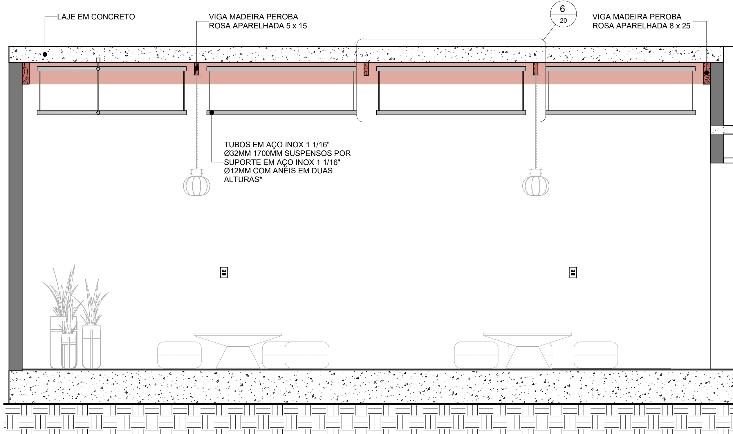
2 CORTE BB - SALÃO PRIVATIVO 1 : 25
