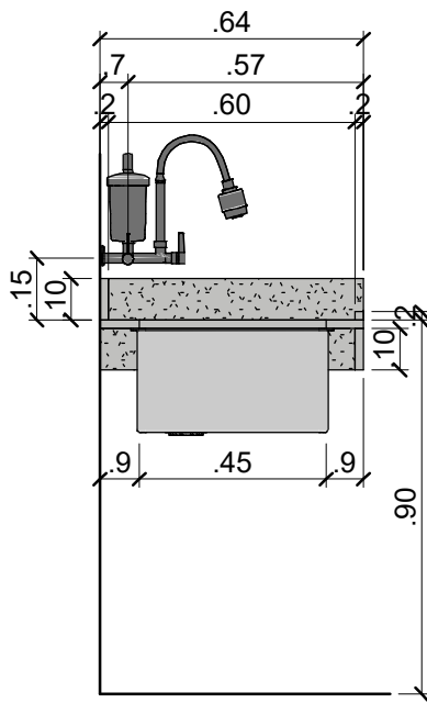
7 BG7: CORTE 1 : 20
