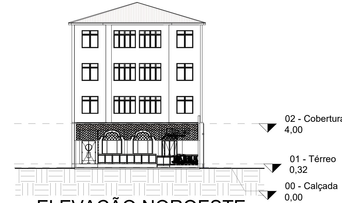
1 ELEVÇÃO NOROESTE 1 : 200
