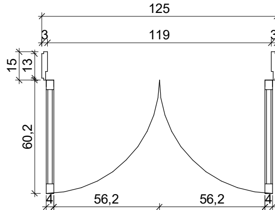
2 P05 - PLANTA 1 : 20
