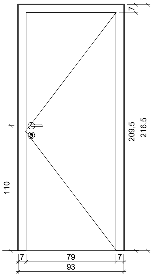
4 P02 - VISTA FRONTAL 1 : 20
