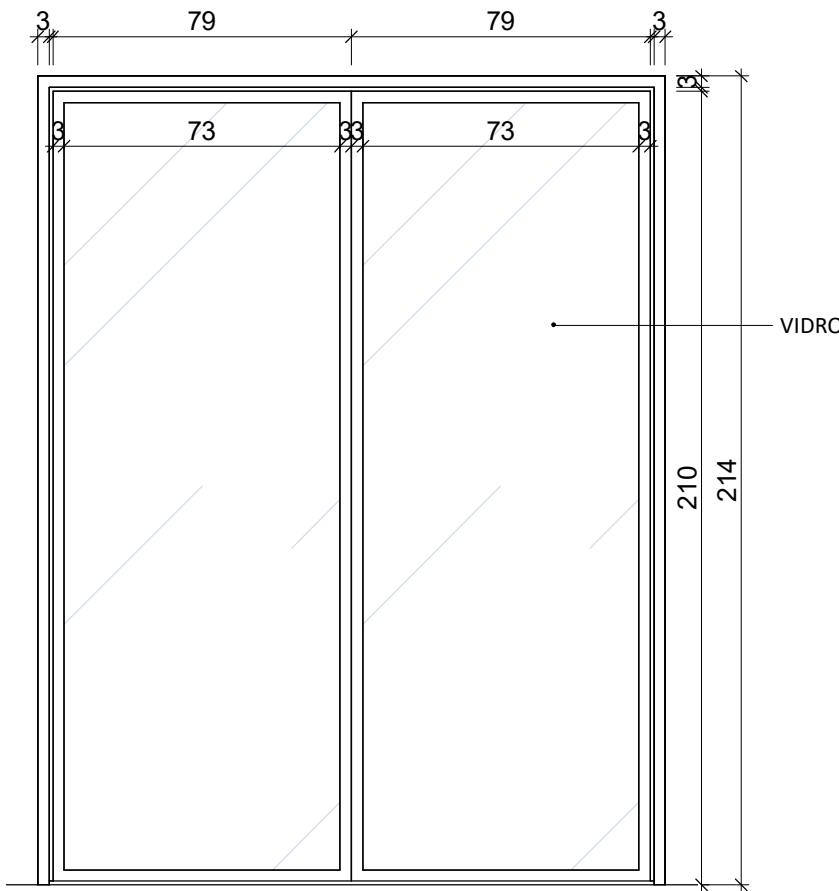
4 P06 - VISTA FRONTAL 1 : 20
