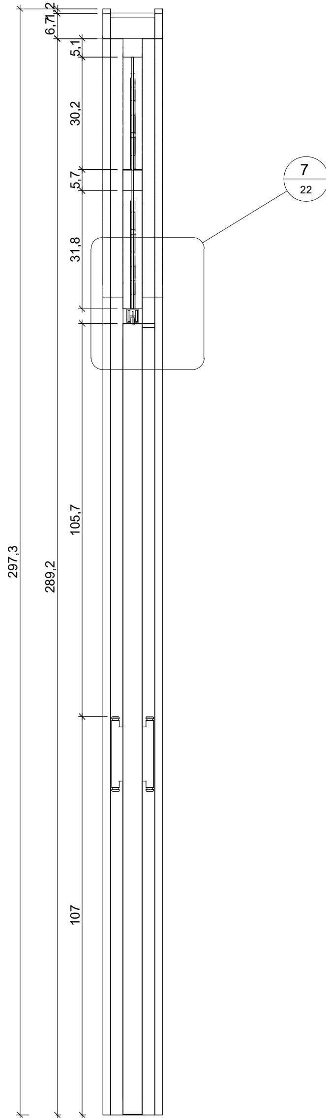
6 CORTE TRANSVERSAL 1 : 10
