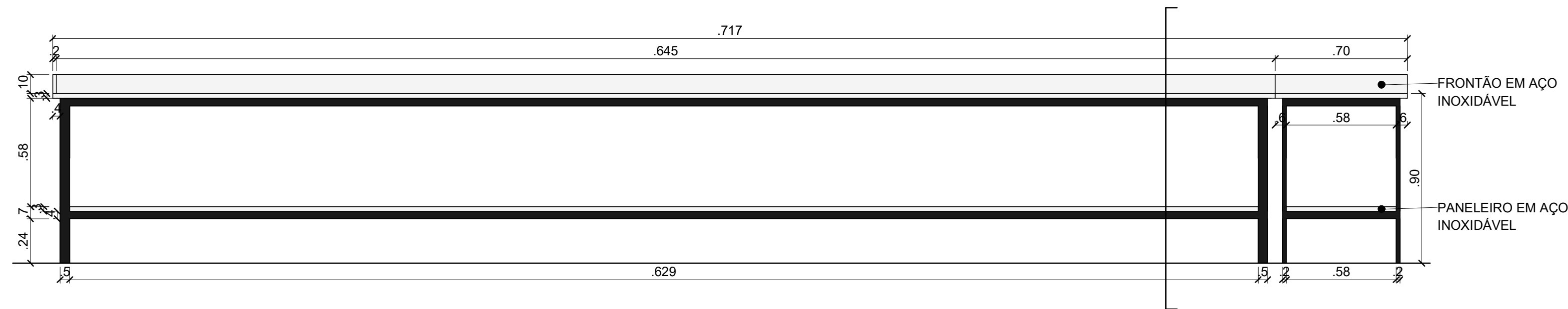
2 BG5: VISTA FRONTAL 1 : 20
