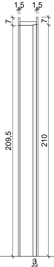
6 P02 - CORTE 1 : 20
