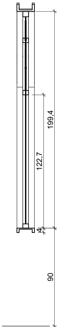
9 J01 - CORTE 1 : 20
