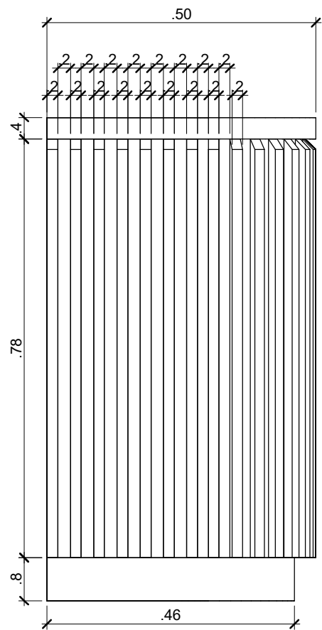
3 ELEVÇÃO LATERAL 1 : 10
