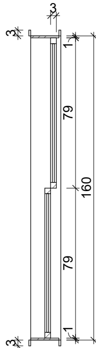
5 P06 - PLANTA 1 : 20
