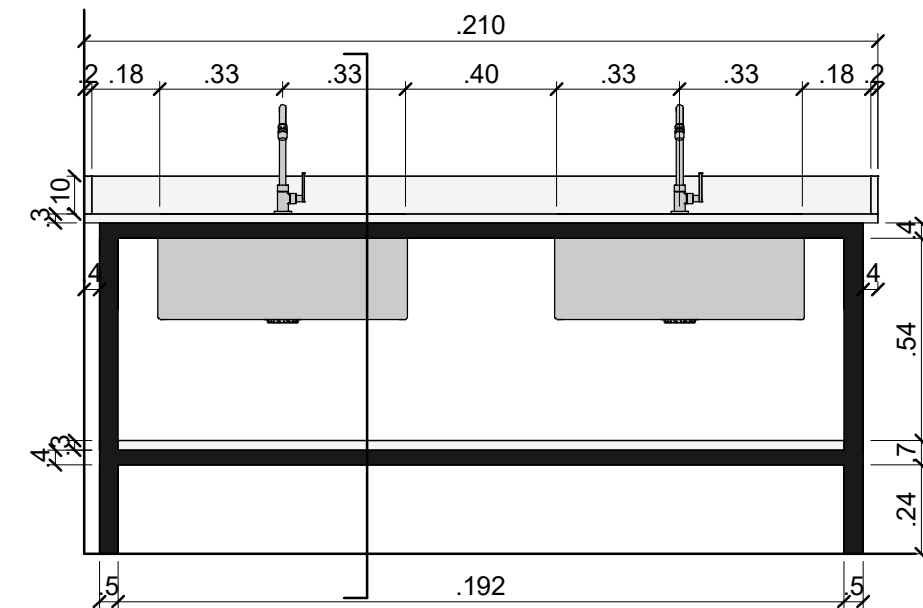
6 BG4: VISTA FRONTAL 1 : 20
