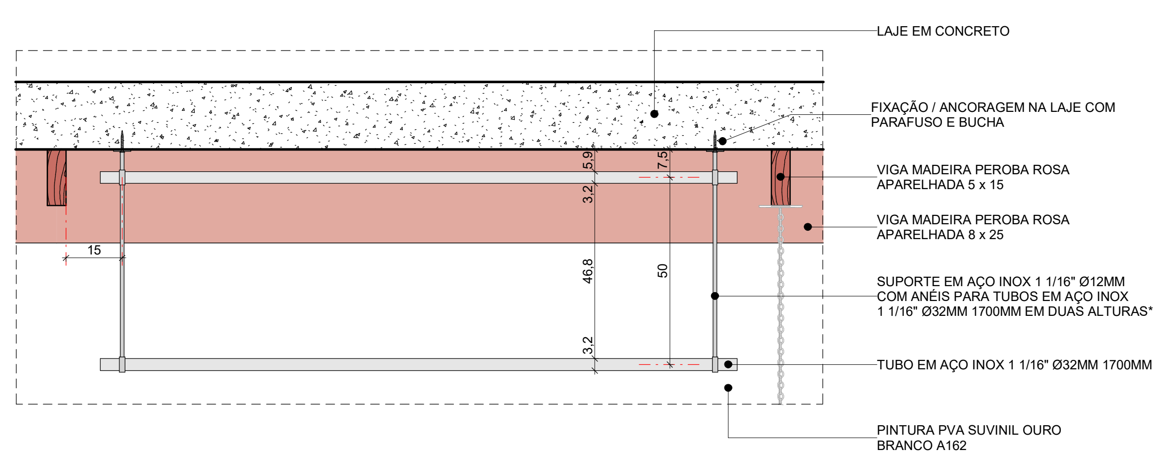
6 AMPLIAÇÃO 02 1 : 10
