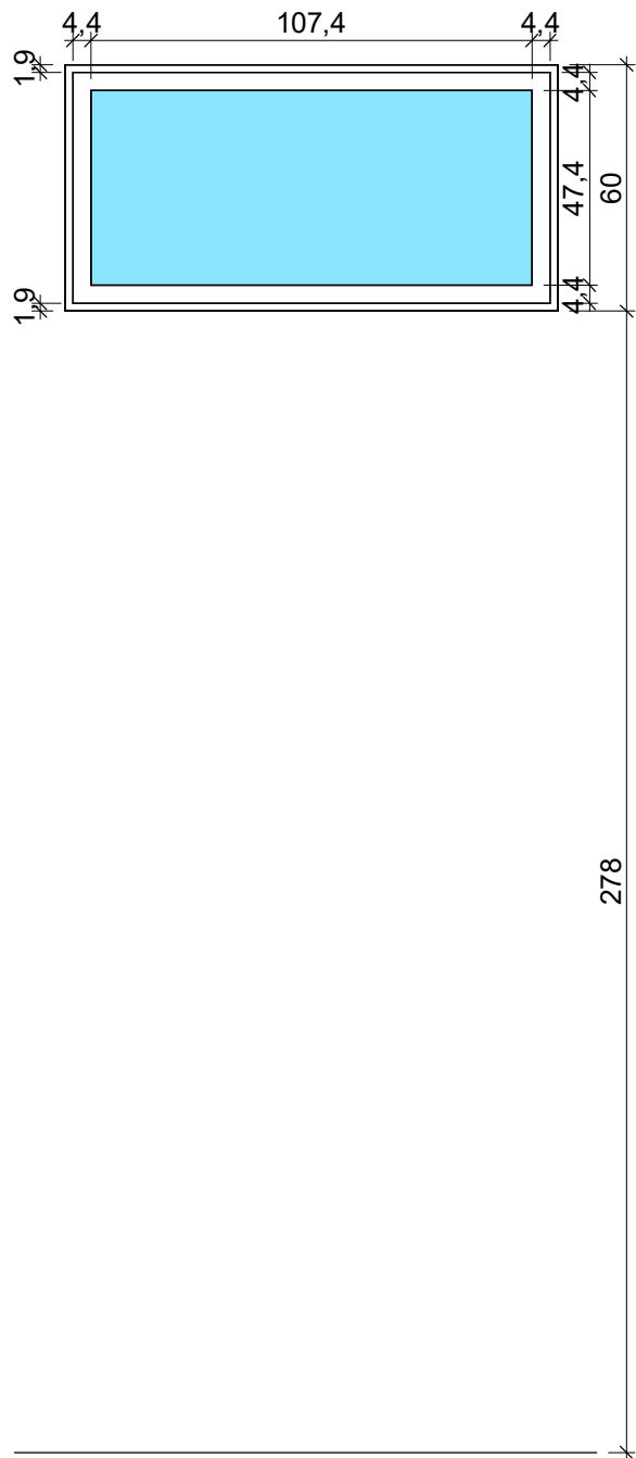
10 J02 - VISTA FRONTAL 1 : 20
