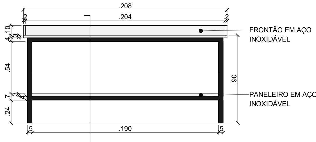
2 BG6: VISTA FRONTAL 1 : 20
