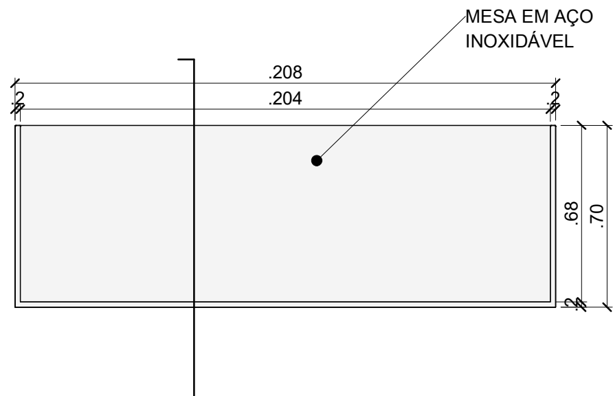
1 BG6: PLANTA 1 : 20
