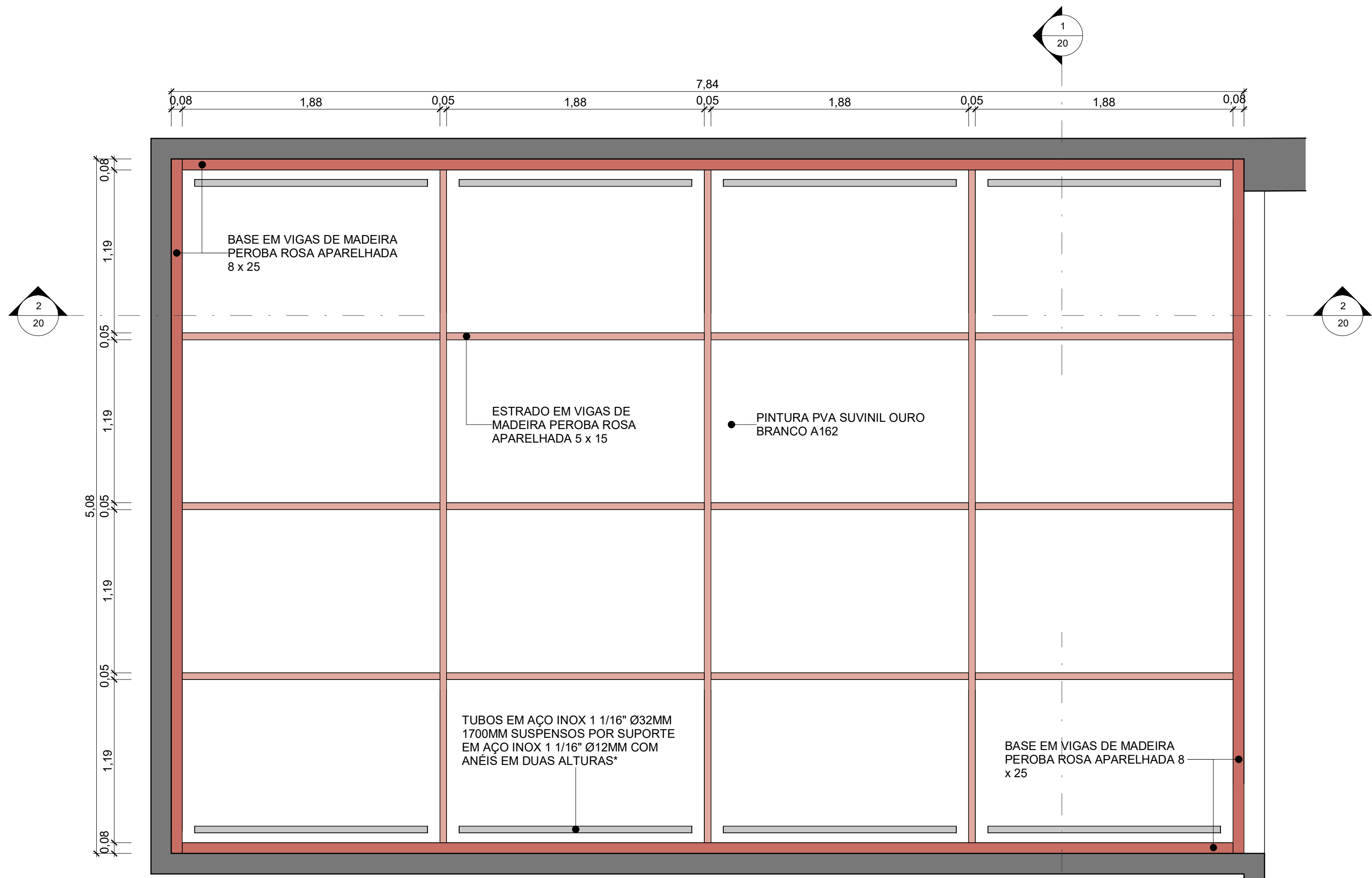
1 TETO - SALÃO PRIVATIVO 1 : 25
