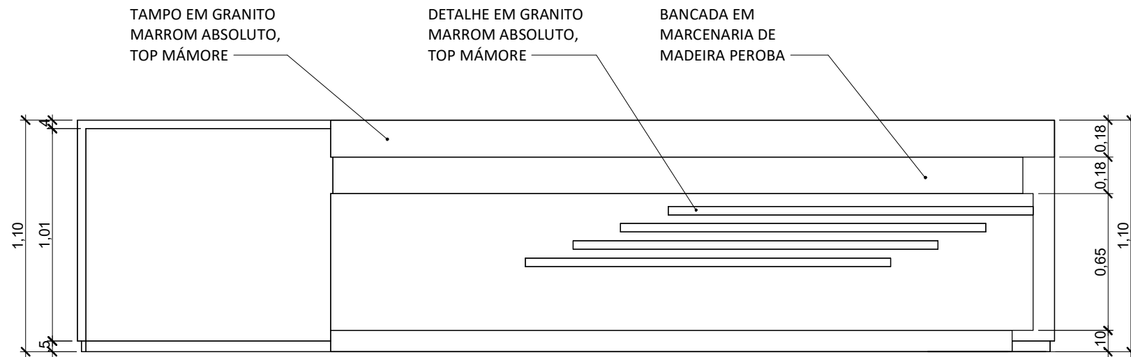
2 ELEVAÇÃO FRONTAL 1 : 25
