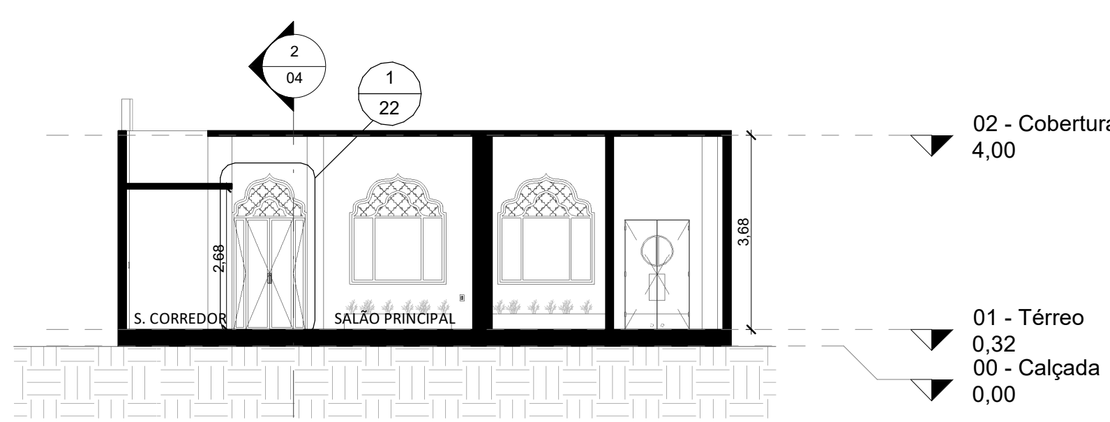
4 CORTE EE 1 : 100
