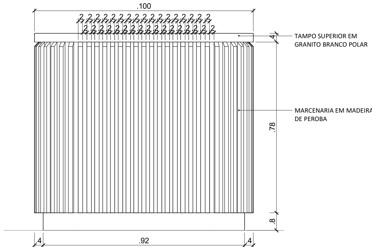
2 ELEVÇÃO FRONTAL 1 : 10
