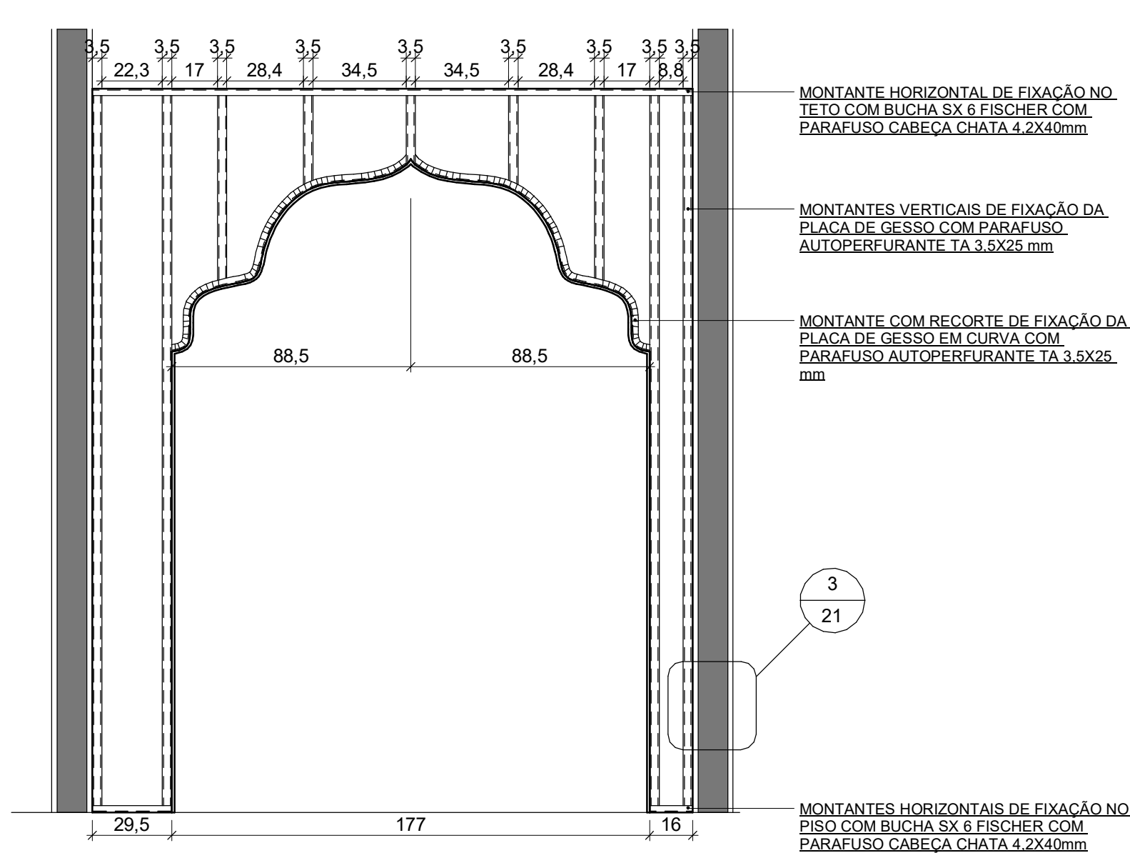
2 DETALHE A - PAREDE DRYWALL DISTÂNCIAS MONTANTES 1 : 20
