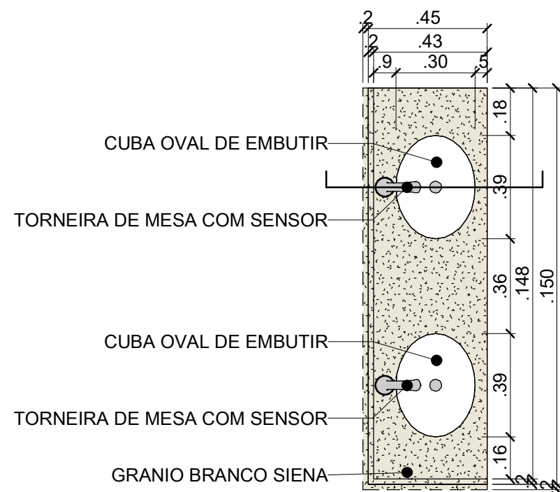
5 BG2: PLANTA 1 : 20
