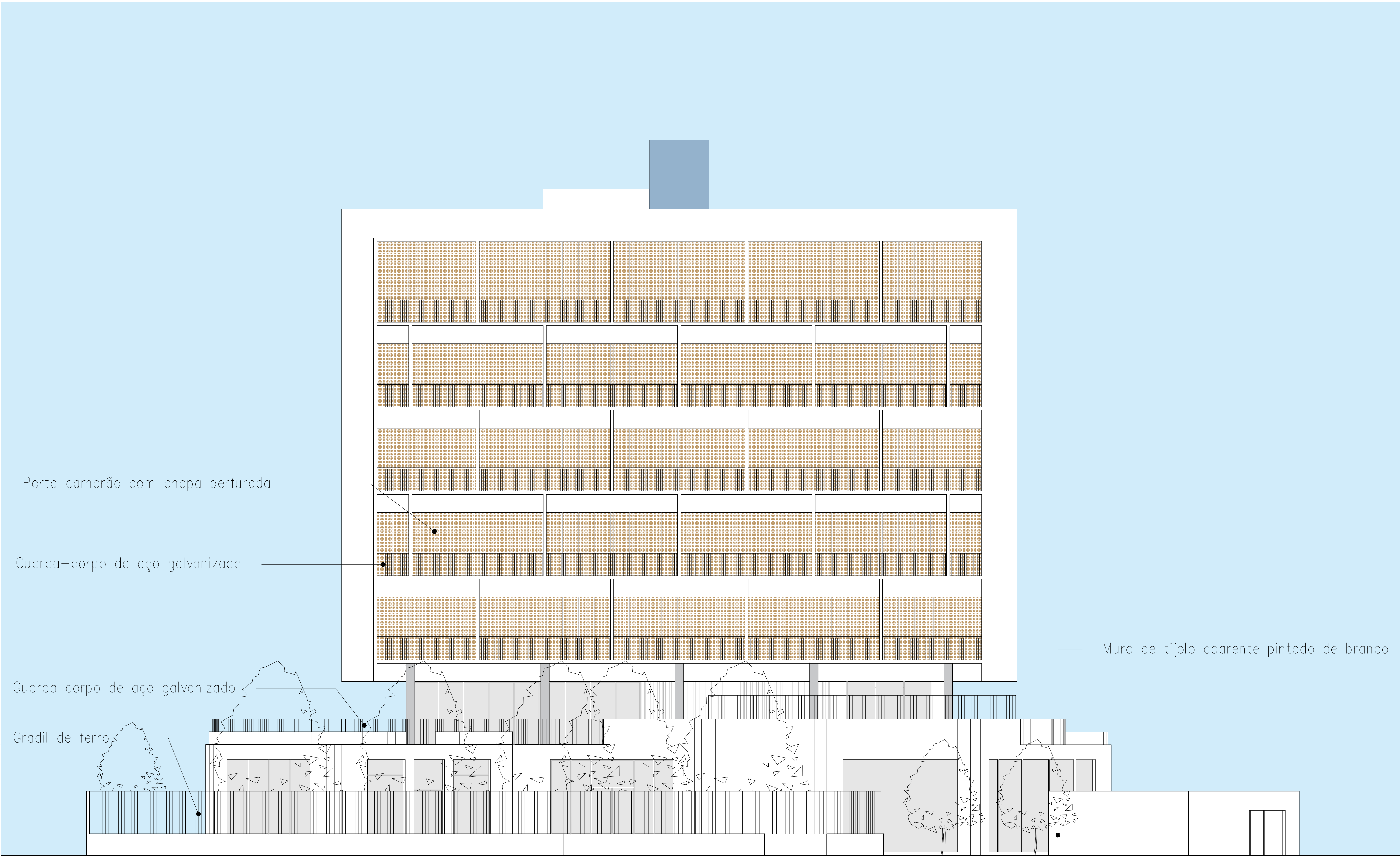
1 Fachada Oeste Esc. 1/100
