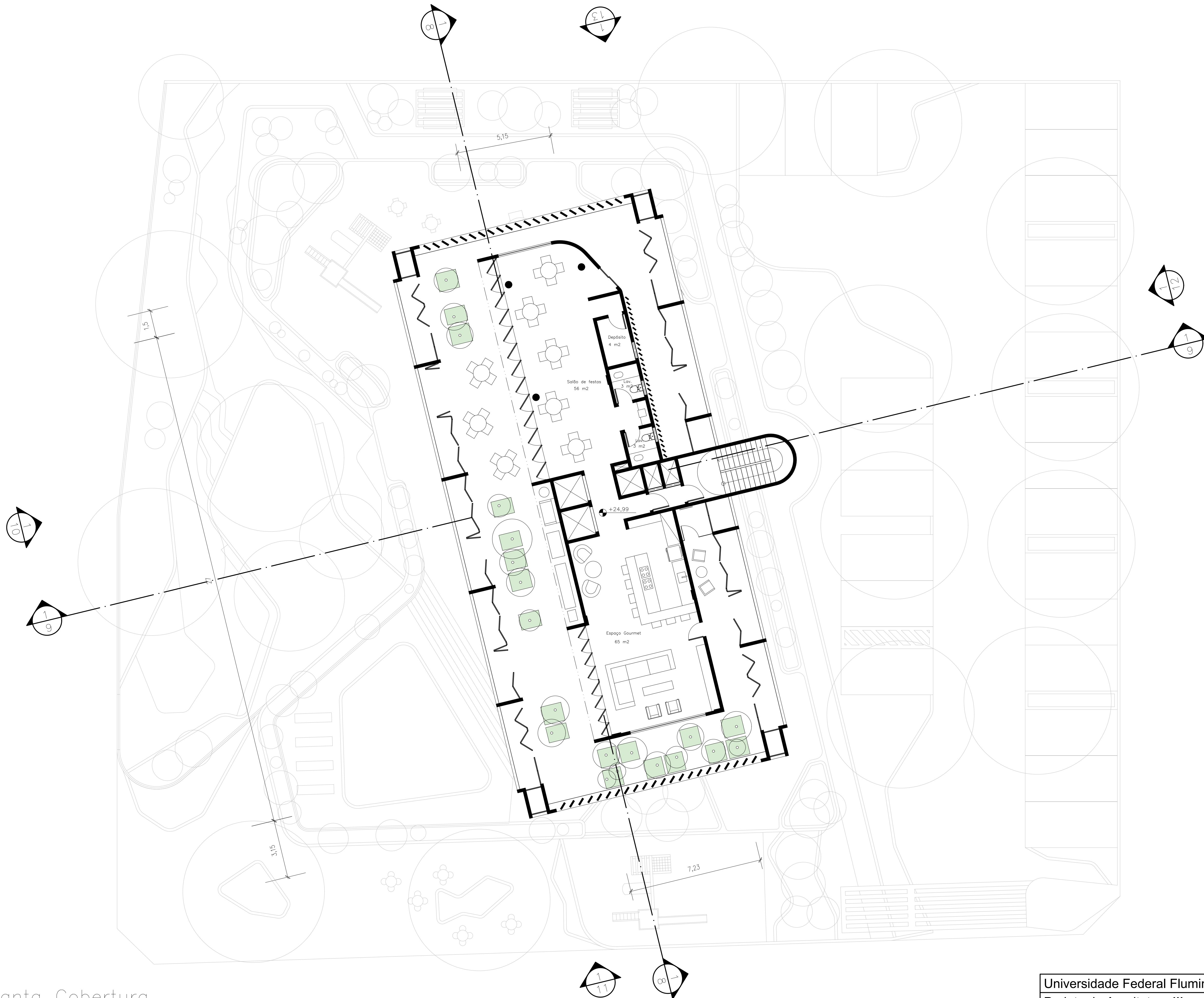
1 Planta Cobertura Esc. 1/100
