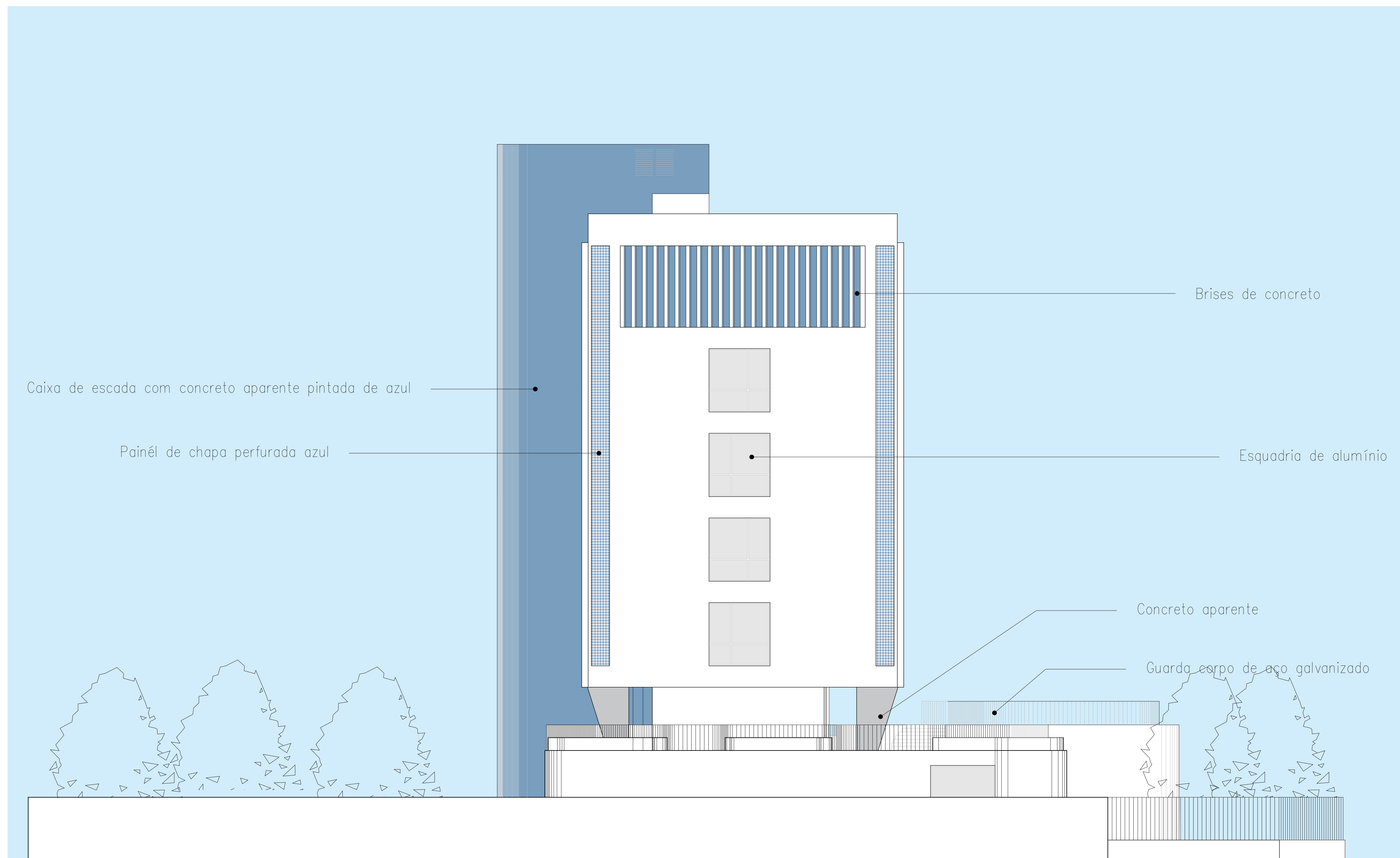
1 Fachada Norte Esc. 1/100
